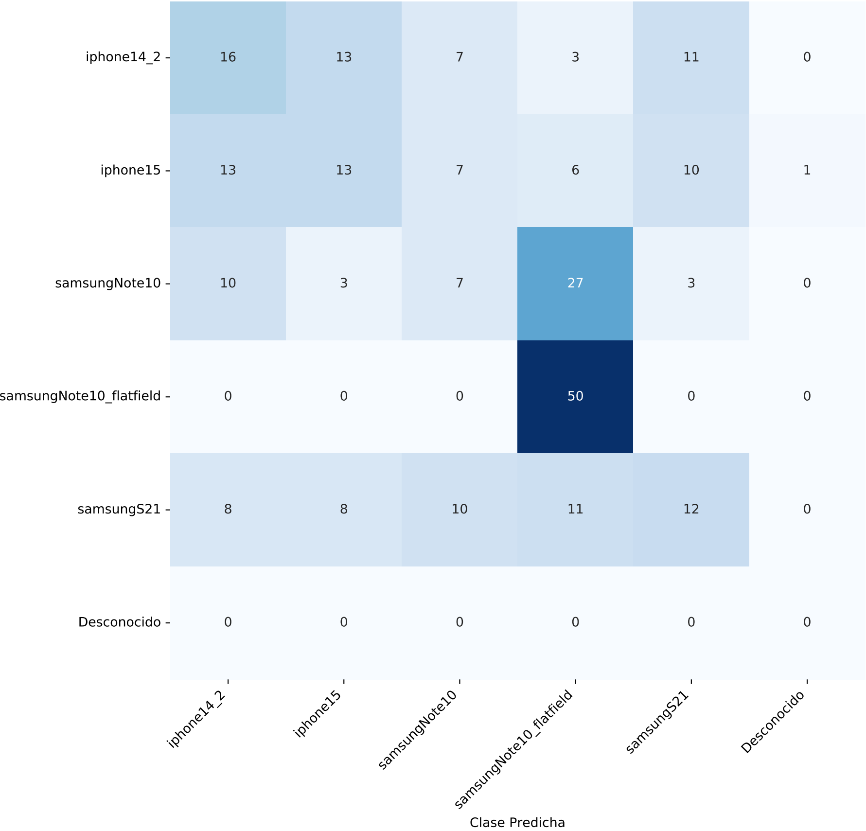
Matriz de Confusión - PRNU_ORIGINALES
