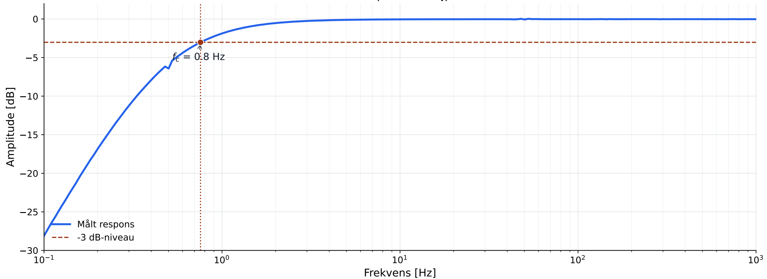
Frekvensrespons for højpasfilter
