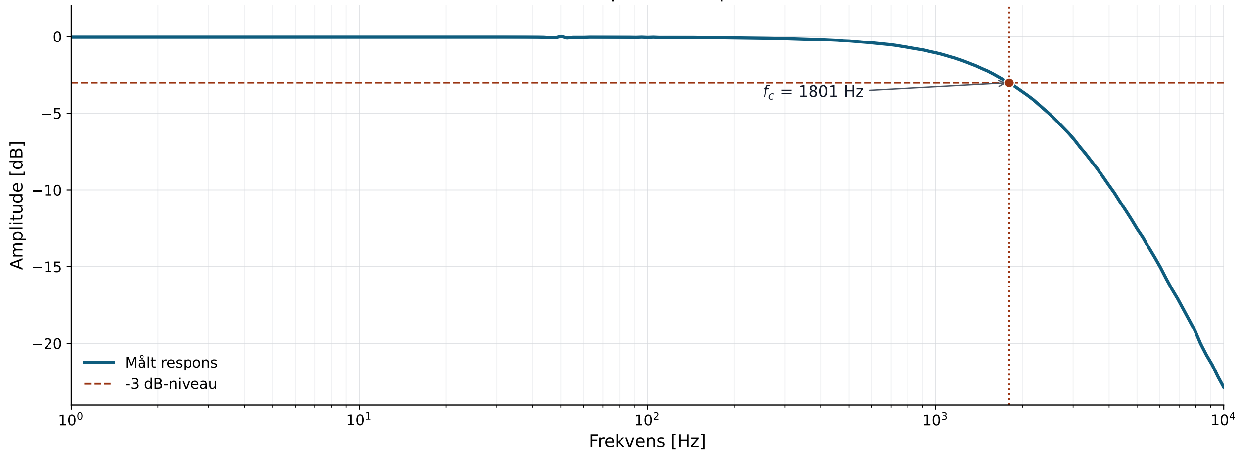
Frekvensrespons for lavpasfilter
