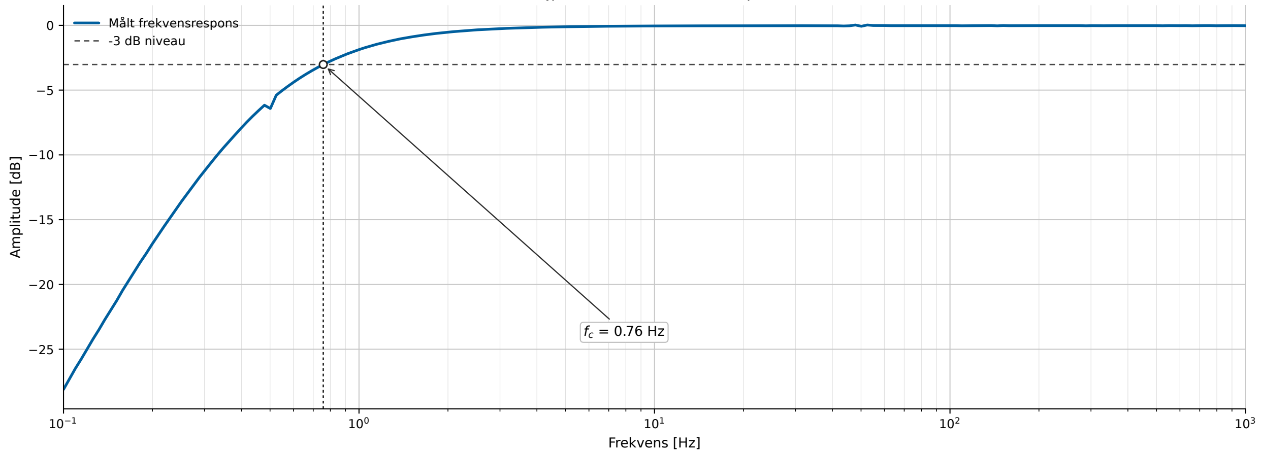
Højpasfilter: målt frekvensrespons
