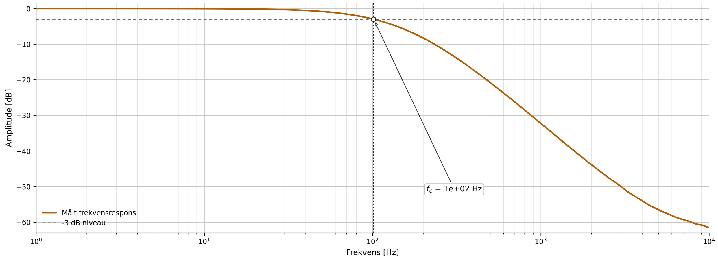
Lavpasfilter: målt frekvensrespons
