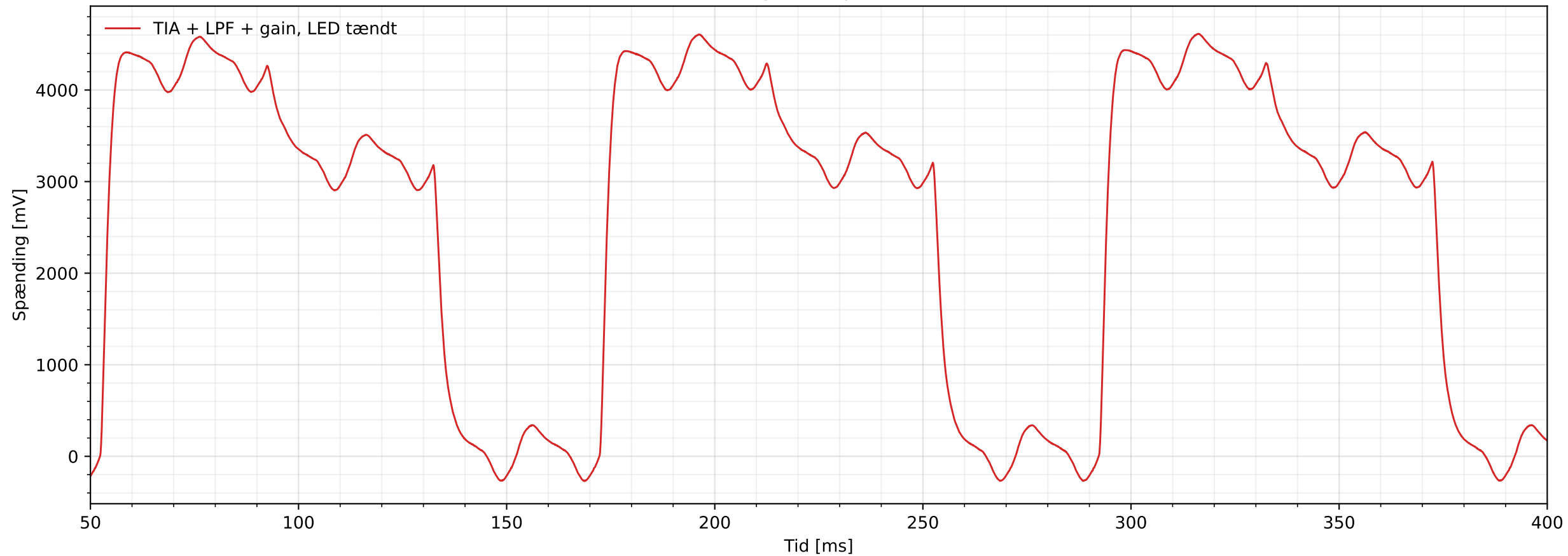
TIA + LPF + gain output - LED tændt
