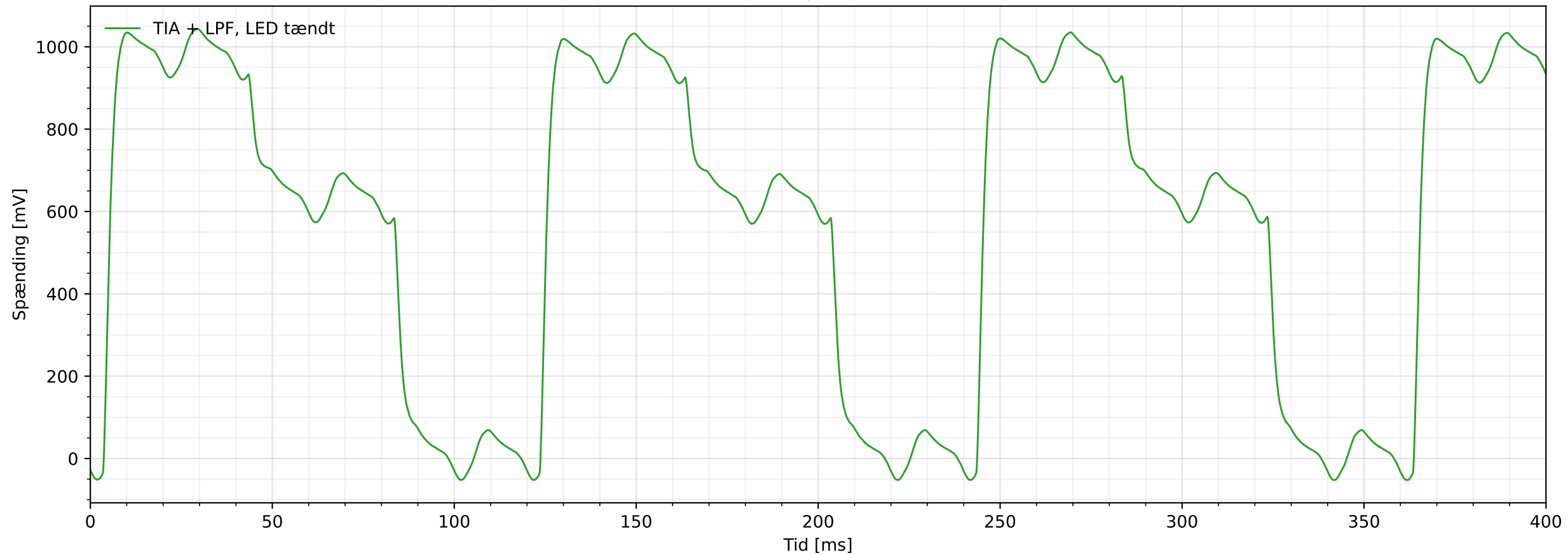
TIA + LPF output - LED tændt
