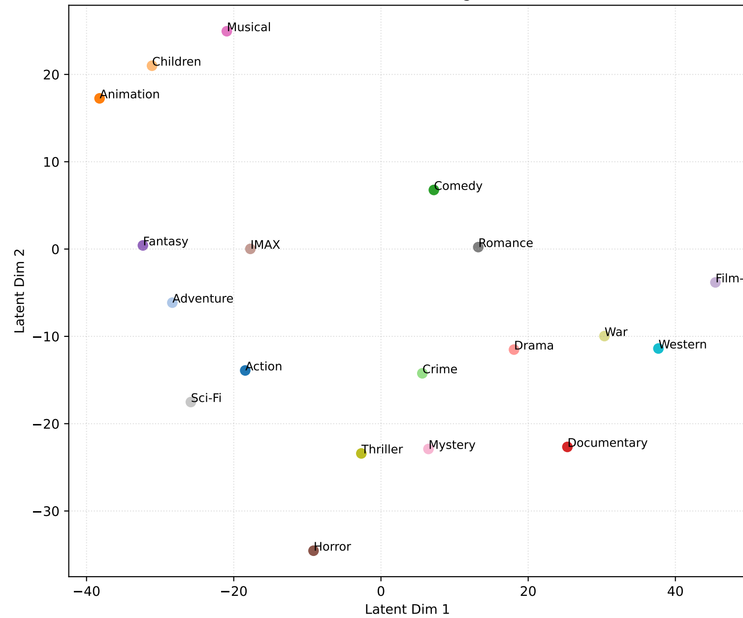
Genre Latent Embeddings (k=10)
