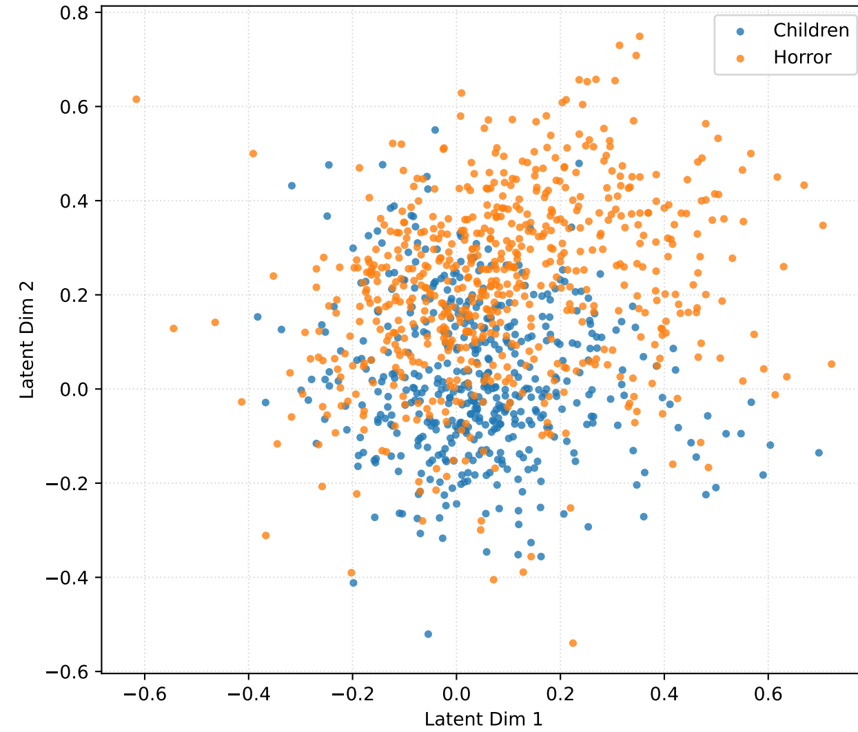
k=10
