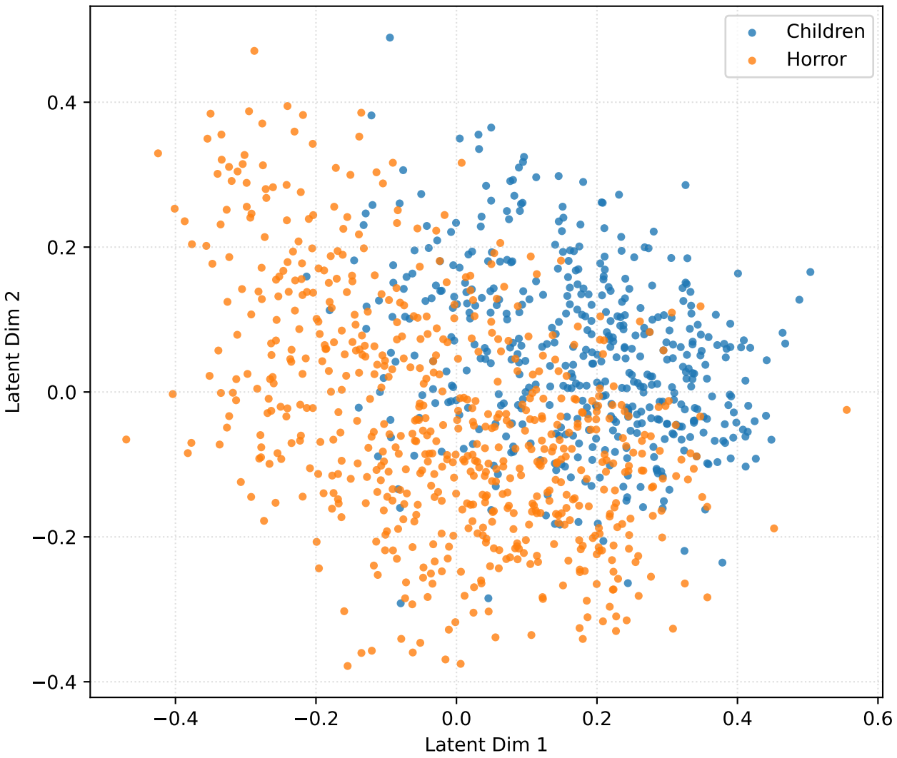
k=2
