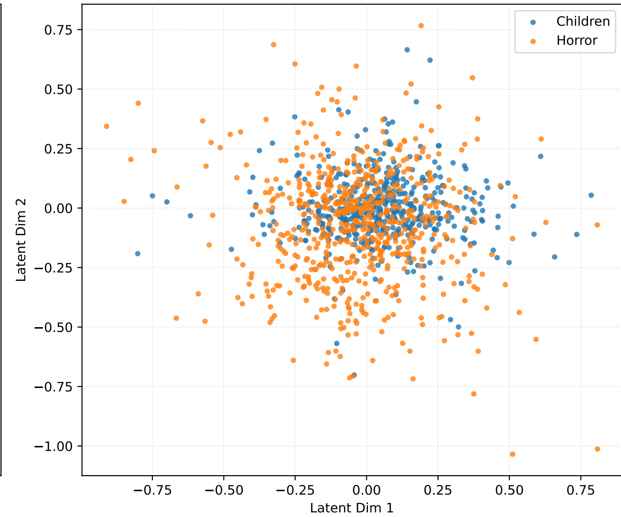
k=20
