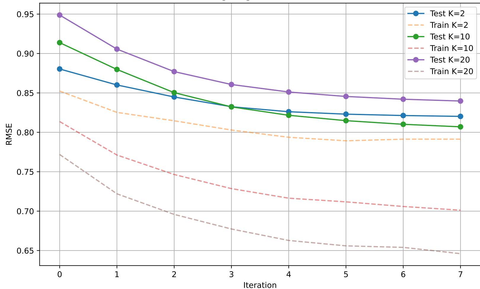
ALS Training Progress for 32m Dataset
