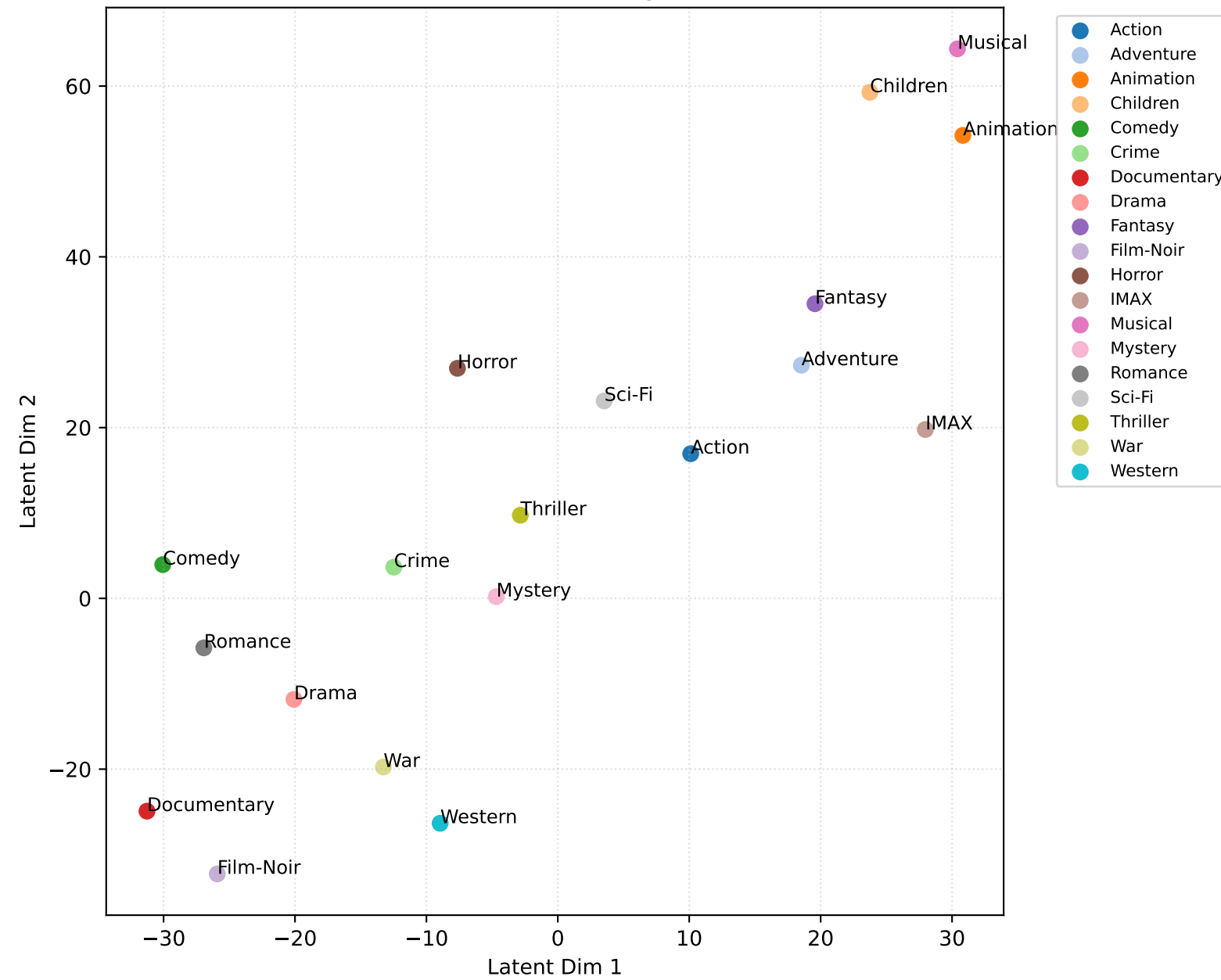
Genre Latent Embeddings (k=10)
