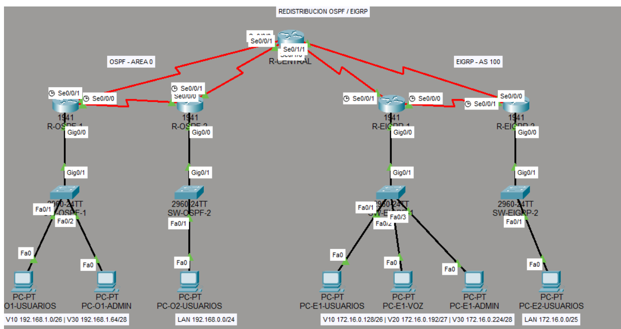
Figura 1: Topologia real construida: cinco routers, seis enlaces seriales, cuatro switches y siete hosts de prueba.
