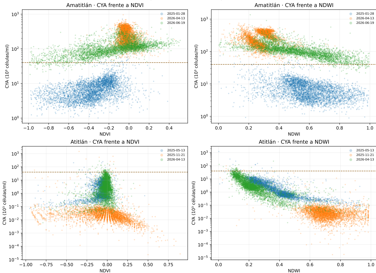
Figura 4: Dispersión entre CYA, NDVI y NDWI en fechas representativas. CYA se muestra en escala logarítmica.
