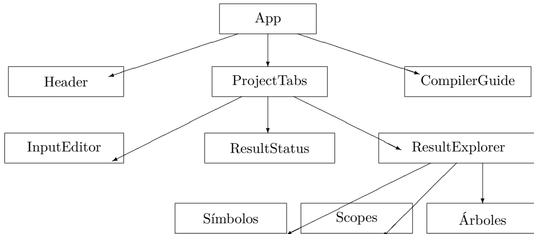
Figura 11.1: Jerarquía simplificada de componentes React.
