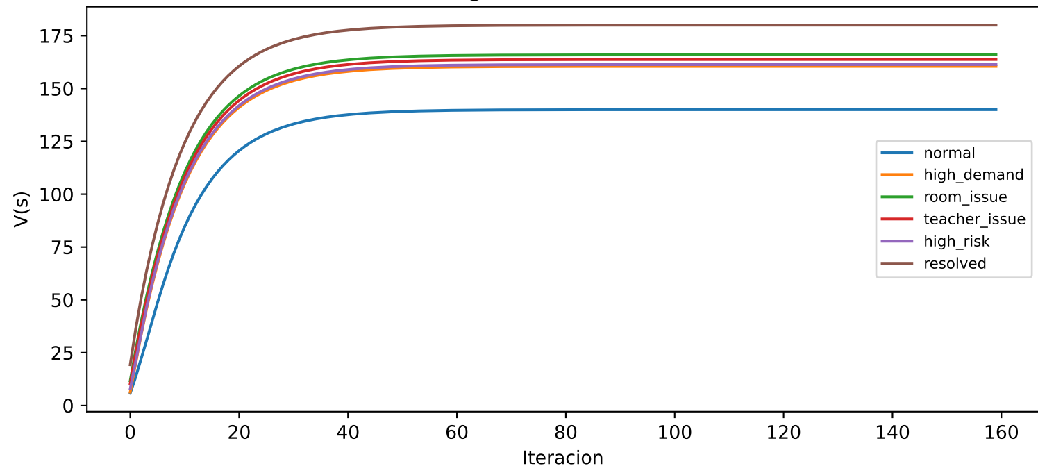
Convergencia Value Iteration
