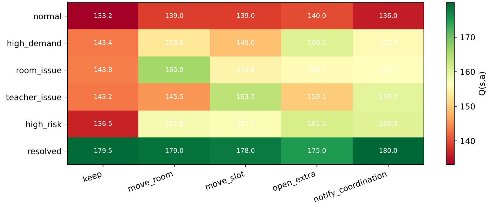
Mapa de calor Q(s,a) — MDP
