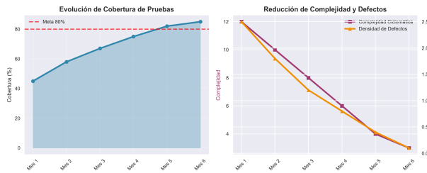
Figura 3: Evolución de métricas de calidad a lo largo del desarrollo del Portal
