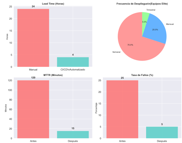
Figura 4: Métricas DORA: Lead Time, MTTR y Frecuencia de Despliegue
