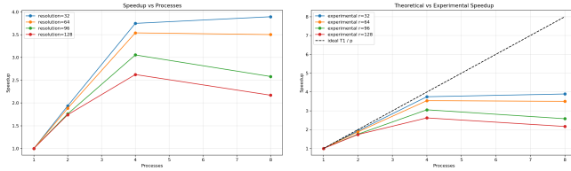
Fig. 2. Speedup medido por cantidad de procesos y comparacion contra la tendencia ideal T_1/p .
