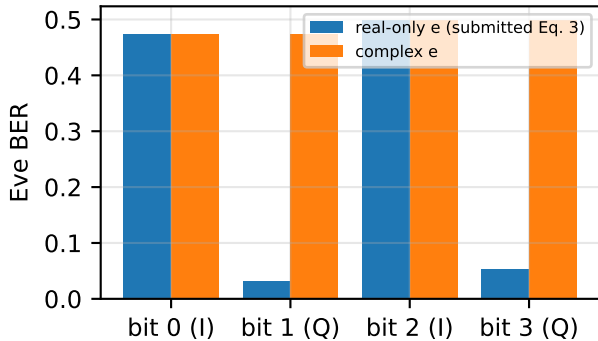
(a) Eve per bit, UMi, 160 dB
