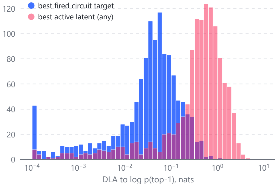
Best DLA per position
