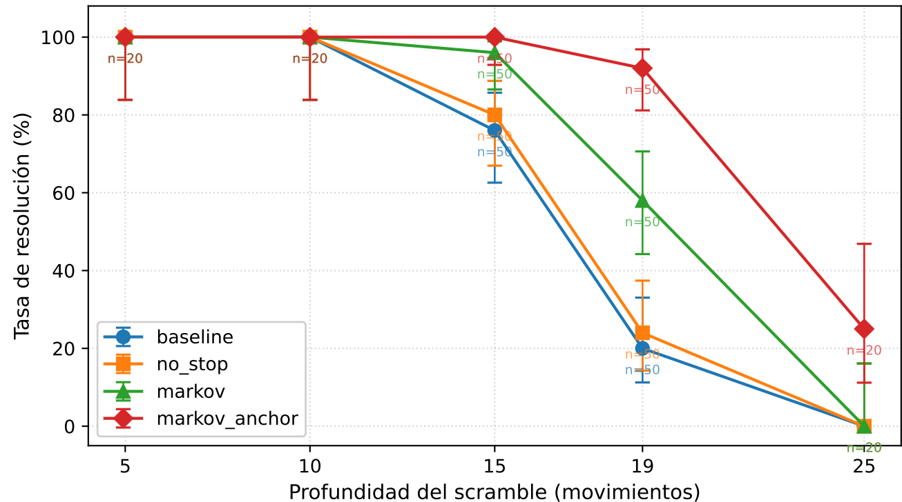
EDA Fuse 3x3x3: tasa de resolución vs profundidad (barras = IC 95% Wilson)
