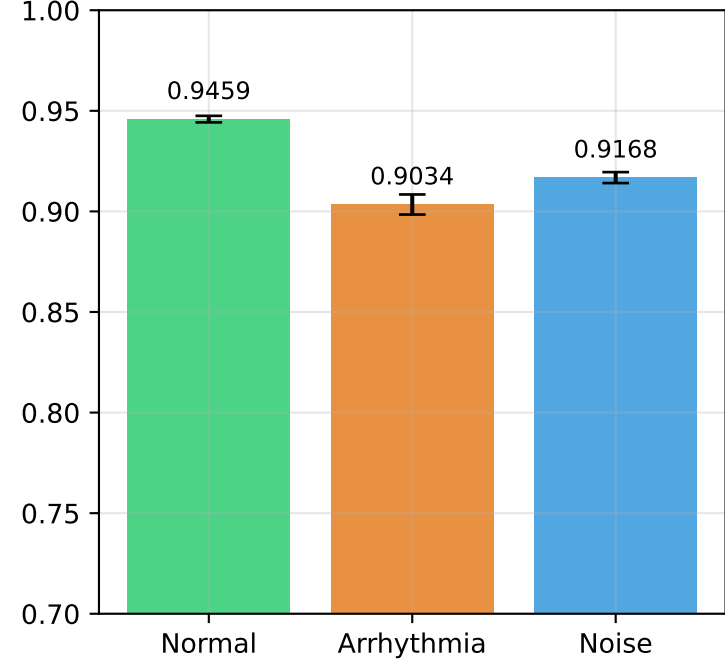
B. Mean Per-Class F1 ( \pm SD)
