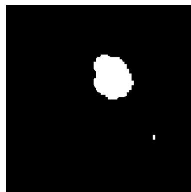
RoCU-Net
