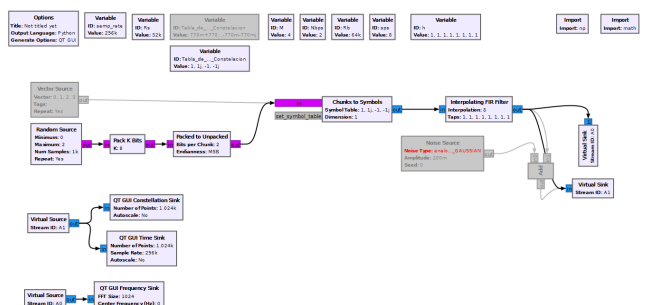
Figura 4. Flujo de bloques de QPSK creado en base al video.
