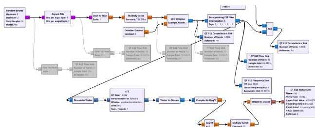
Figura 2 Flujo de bloques de M-PSK modificado para PSD.
