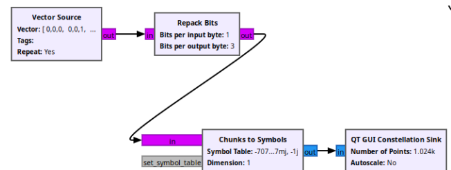
Figura 3. Flujo de bloques modificado, reprogramar tabla de la verdad
