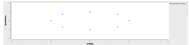
Figura 7. Constelación 8-PSK mediante mapeo directo de símbolos.
