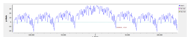
Figura 10. PSD para QPSK.
