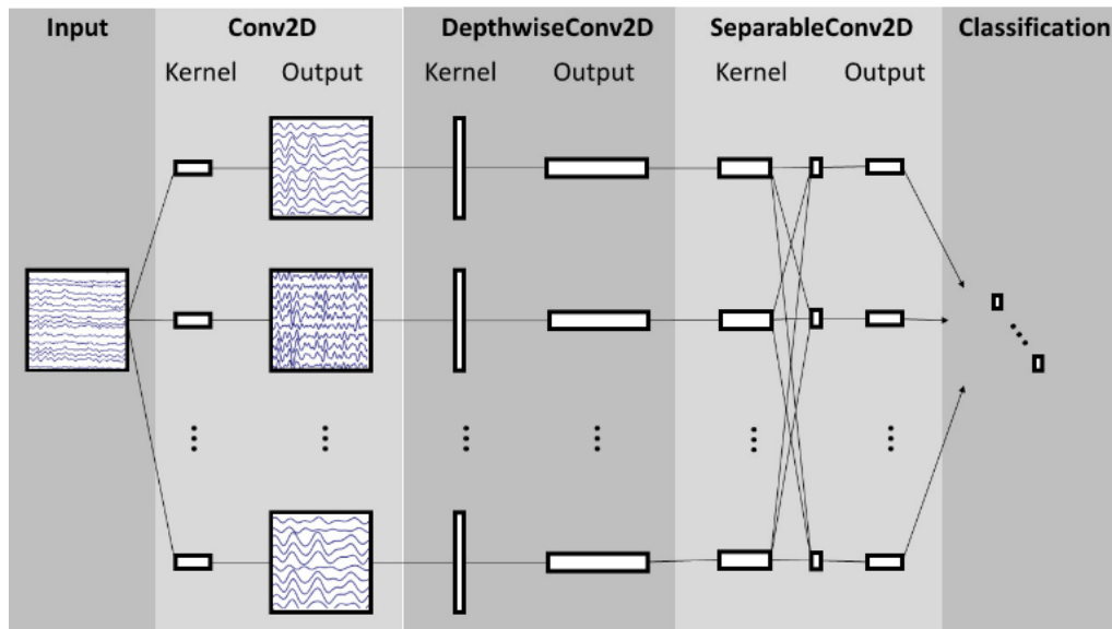
Figura 3.3: Arquitectura de EEGNet. las líneas muestran la conexión entre las capas [50].
