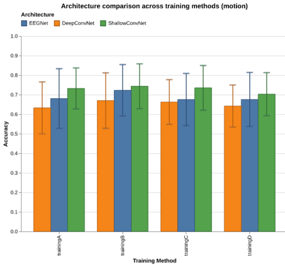
Figura 4.4: Comparación general de las distintas arquitecturas y métodos de entrenamiento en la tarea de movimiento
