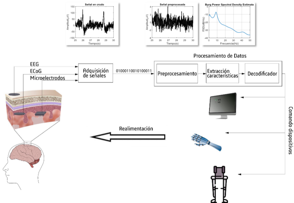
Figura 2.1: Esquema general de una BCI [16]
