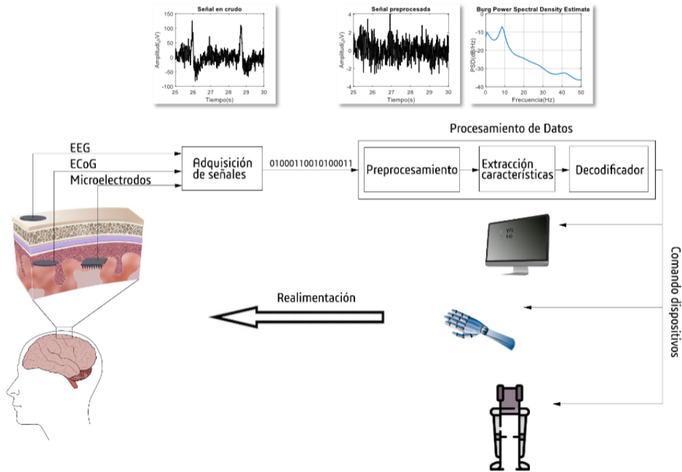
Figura 2.2: Esquema general de una BCI [25]
