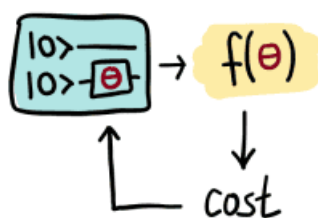
Figura 6.2: Coste de un Circuito Cuántico Variacional, imagen obtenida de: [22]
