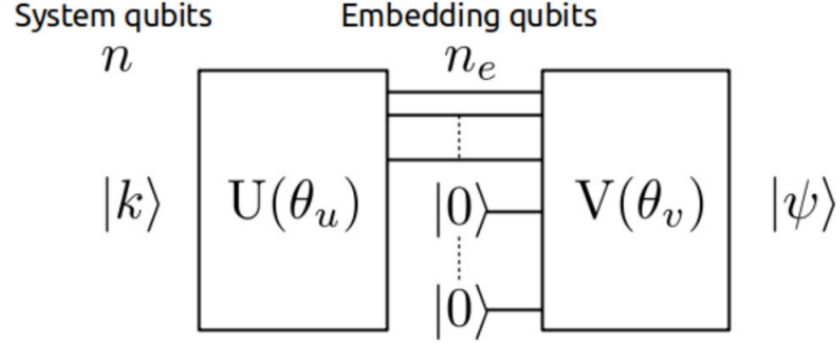
Figura 9.1: Estructura de QWord2Vec. Fuente: [21].
