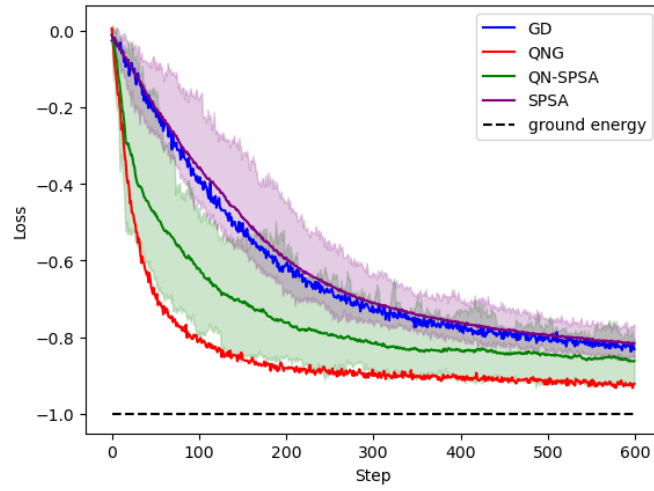
Figura 9.5: Comparativa de los algoritmos de optimización GD, SPSA, QNG y QN-SPSA en términos de convergencia y coste computacional. Fuente: [5].
