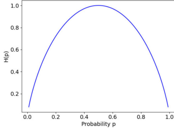
Figura 9.4: Entropía binaria H(p) , donde p denota la probabilidad de error empleada en este estudio. Fuente: [21].
