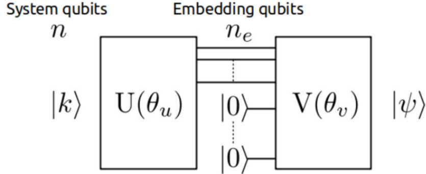
Figura 4.9: Estructura de QWord2Vec . Fuente: [55].
