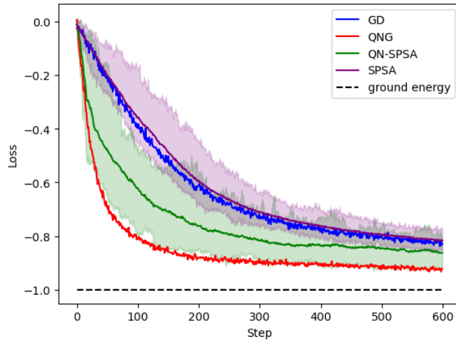
Figura 4.13: Comparativa de los algoritmos de optimización GD, SPSA, QNG y QN-SPSA en términos de convergencia y coste computacional. Fuente: [22].
