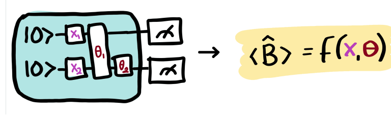
Figura 2.10: Circuito variacional cuántico con parámetros modificables \theta y no modificables x . Imagen obtenida de: [57]
