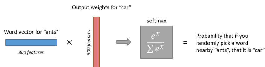
Figura 4.8: Cálculo de la salida de la neurona correspondiente a la palabra car en la capa softmax del modelo Skip-gram. Fuente: [48].
