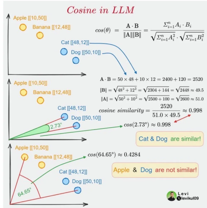
Figura 3.2: Ejemplo visual de la representación de vectores y su cercanía empleando la similitud coseno. Fuente: [42].
