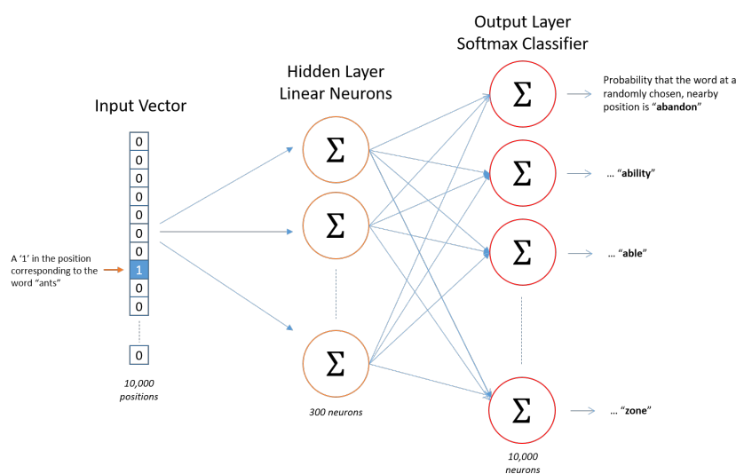
Figura 4.5: Arquitectura de la red neuronal del modelo Skip-gram. Fuente: [48].
