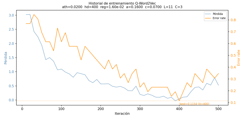
Figura 5.9: Evolución de la función de pérdida (eje izquierdo) y del error rate (eje derecho) durante el entrenamiento de QWord2Vec sobre el corpus ampliado.
