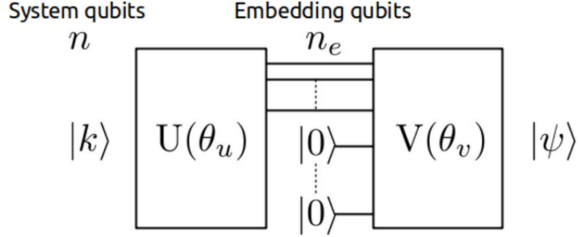
Figura 9.1: Estructura de QWord2Vec. Fuente: [28].
