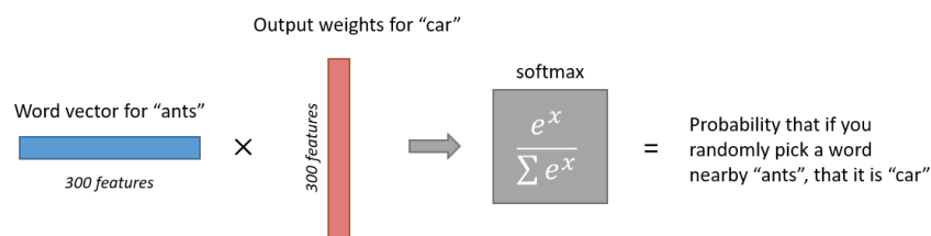
Figura 8.8: Cálculo de la salida de la neurona correspondiente a la palabra car en la capa softmax del modelo Skip-gram. Fuente: [24].
