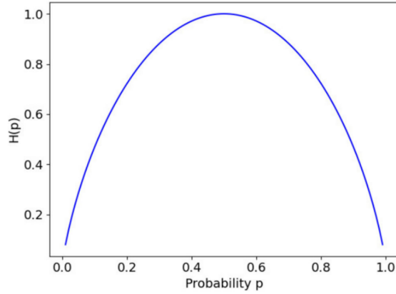
Figura 9.4: Entropía binaria H(p) , donde p denota la probabilidad de error empleada en este estudio. Fuente: [28].
