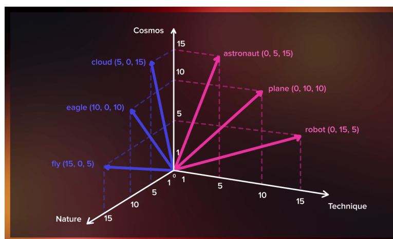
Figura 8.2: Representación vectorial de palabras en el espacio latente generado por Word2Vec. Fuente: [23].
