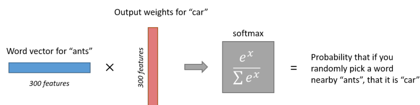
Figura 4.8: Cálculo de la salida de la neurona correspondiente a la palabra car en la capa softmax del modelo Skip-gram. Fuente: [40].
