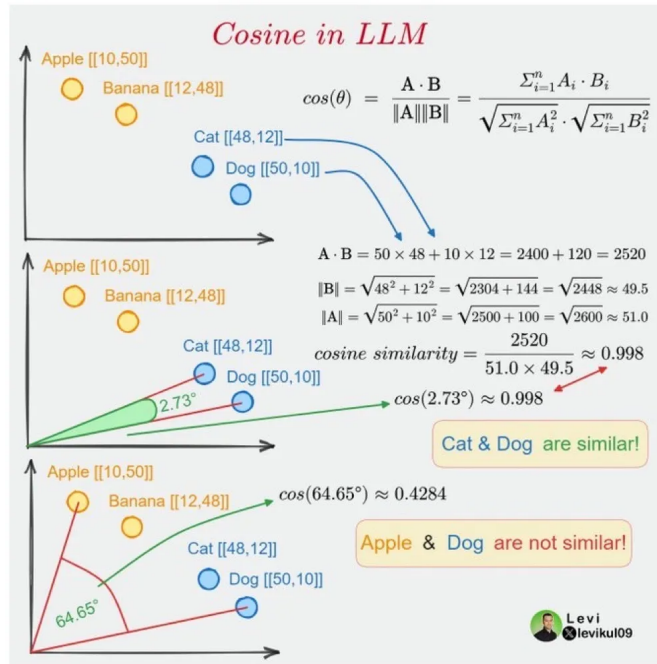
Figura 3.4: Ejemplo visual de la representación de vectores y su cercanía empleando la similitud coseno. Fuente: [35].
