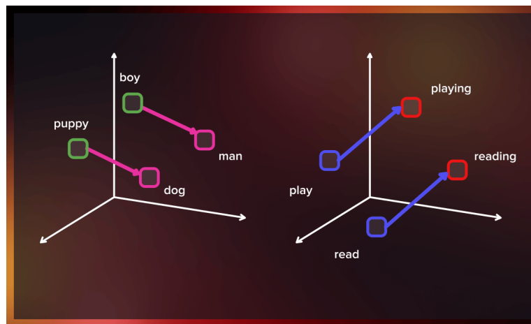
Figura 4.3: Representación geométrica de las similitudes semánticas entre palabras en el espacio vectorial de Word2Vec. Fuente: [38].
