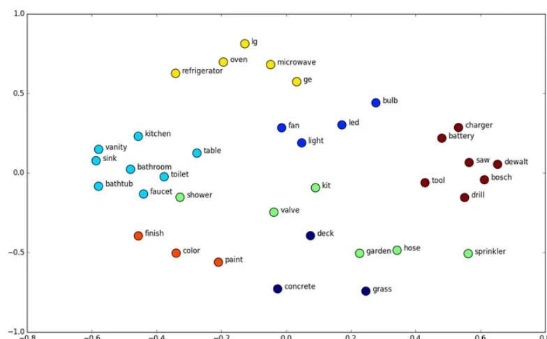
Figura 3.2: Representación visual de un modelo basado en predicciones para generar embeddings de palabras. Fuente: [45].
