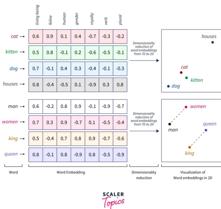
Figura 3.3: Representación visual de un modelo basado en conteos para generar embeddings de palabras. Fuente: [39].
