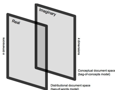
Figura 3.5: Esquema del espacio documental complejo vectorial unificando la semántica distribucional y referencial en el espacio de Hilbert. Fuente: [80].
