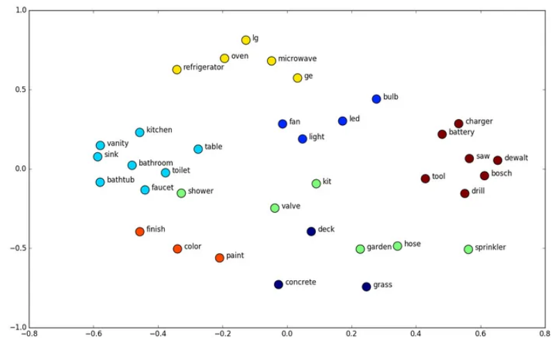
Figura 3.4: Representación visual de un modelo basado en predicciones para generar embeddings de palabras a partir de los pesos de una red neuronal. Fuente: [46].
