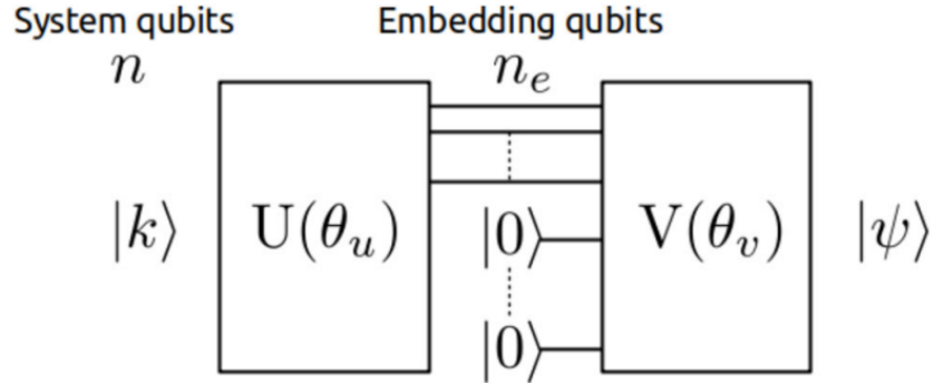
Figura 4.9: Estructura de QWord2Vec . Fuente: [48].
