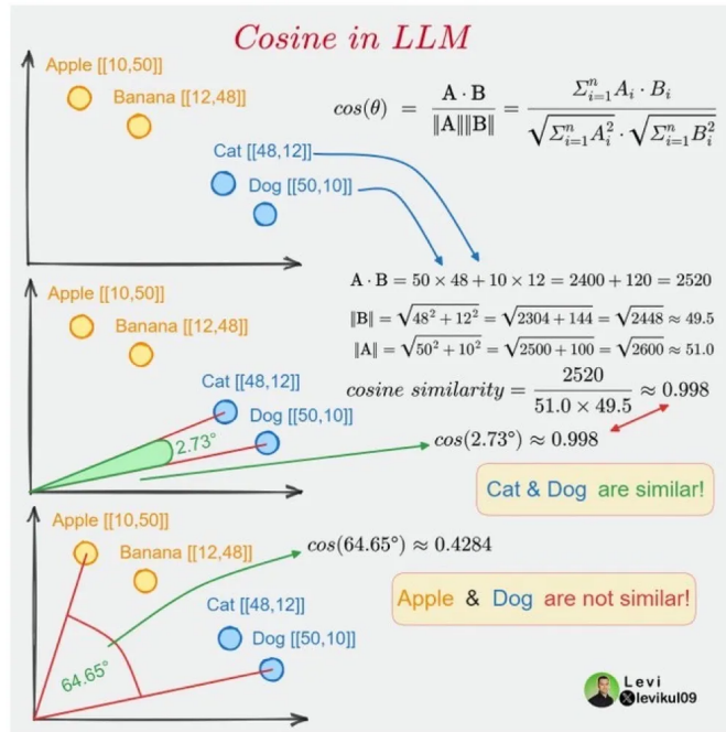
Figura 3.2: Ejemplo visual de la representación de vectores y su cercanía empleando la similitud coseno. Fuente: [36].
