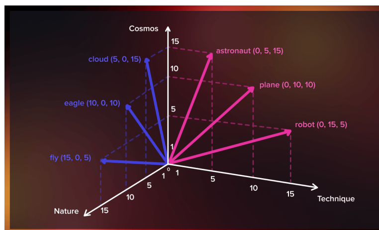
Figura 4.2: Representación vectorial de palabras en el espacio latente generado por Word2Vec. Fuente: [39].
