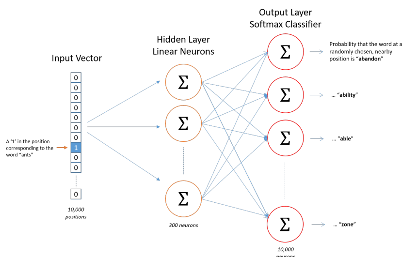
Figura 4.5: Arquitectura de la red neuronal del modelo Skip-gram. Fuente: [41].
