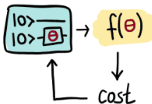
Figura 2.9: Coste de un Circuito Cuántico Variacional, imagen obtenida de: [51]
