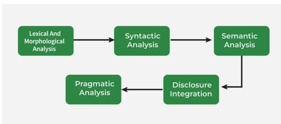
Figura 2.1: Esquema de las fases del PLN. Extraído de [27].
