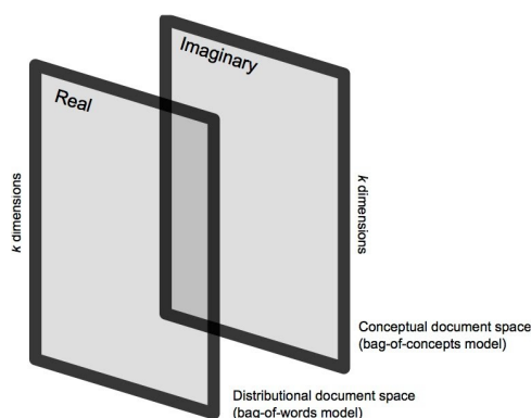
Figura 3.5: Esquema del espacio documental complejo vectorial unificando la semántica distribucional y referencial en el espacio de Hilbert. Fuente: [96].
