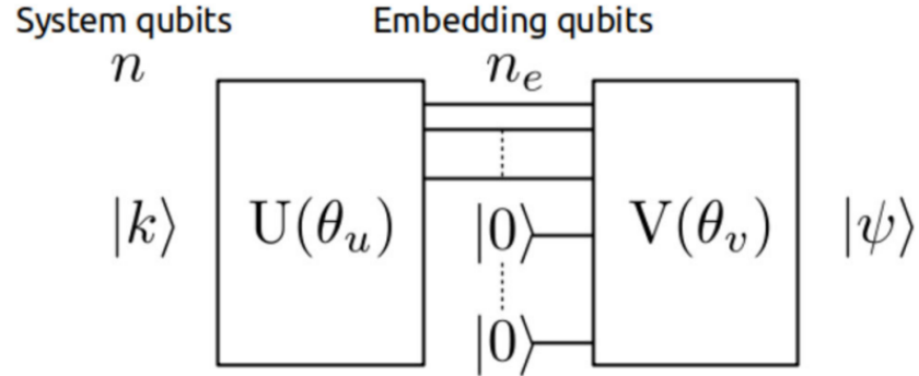
Figura 4.9: Estructura de QWord2Vec . Fuente: [58].
