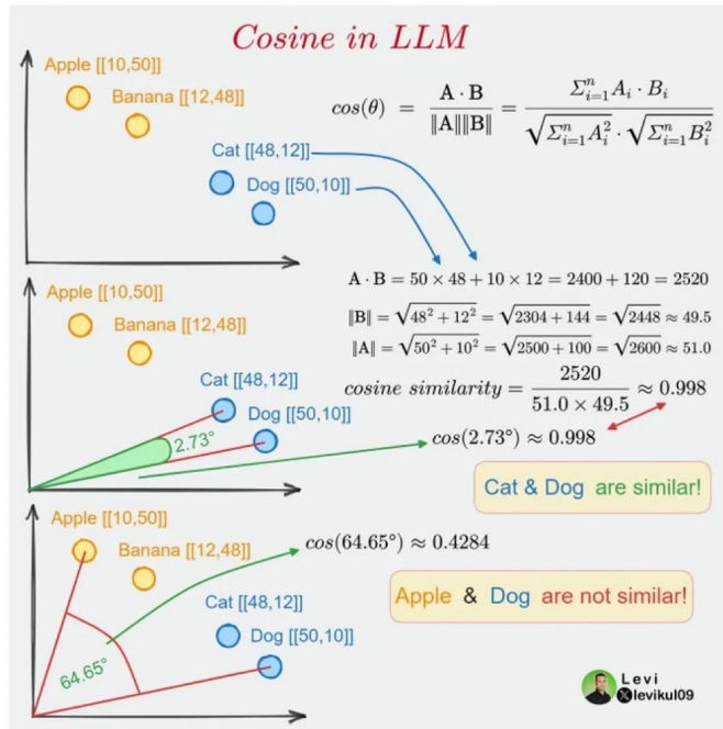
Figura 3.2: Ejemplo visual de la representación de vectores y su cercanía empleando la similitud coseno. Fuente: [44].
