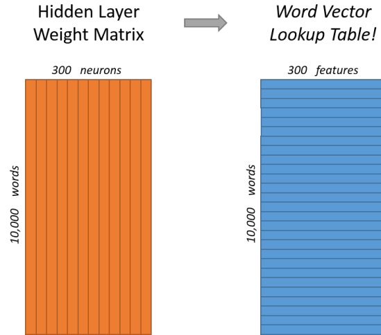
Figura 4.6: Matriz de pesos de la capa oculta del modelo Skip-gram: 10.000 filas (una por palabra del vocabulario) y 300 columnas (una por neurona oculta). Cada fila constituye el vector de representación de su palabra correspondiente. Fuente: [50].
