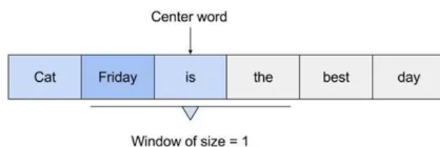
Figura 5.1: Ilustración del parámetro window en Skip-Gram : distancia máxima desde la palabra central hasta las palabras de contexto consideradas. Fuente: [2].
