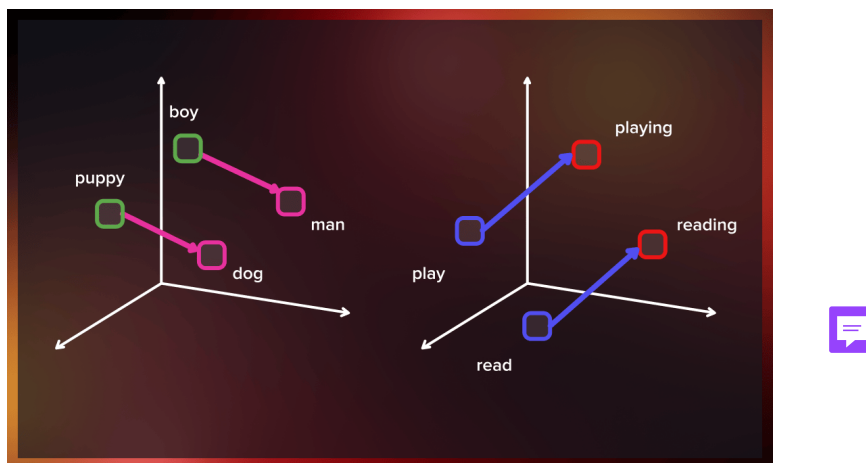
Figura 8.3: Representación geométrica de las similitudes semánticas entre palabras en el espacio vectorial de Word2Vec. Fuente: [20].
