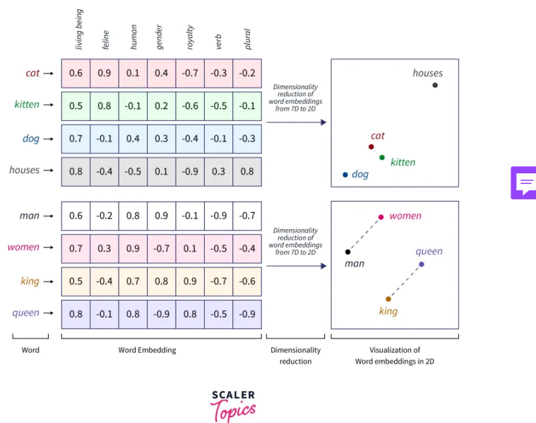
Figura 7.3: Representación visual de un modelo basado en conteos para generar embeddings de palabras. Fuente: https://www.scaler.com/topics/tensorflow/tensorflow-word-embeddings/ .
