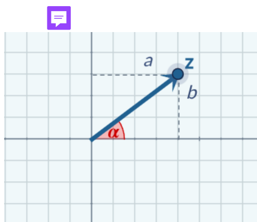
Figura 2.3: Gráfica de la forma polar de un número complejo
