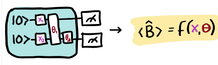
Figura 5.3: Circuito variacional cuántico con parámetros modificables x y no modificables \theta . Imagen obtenida de: [30]
