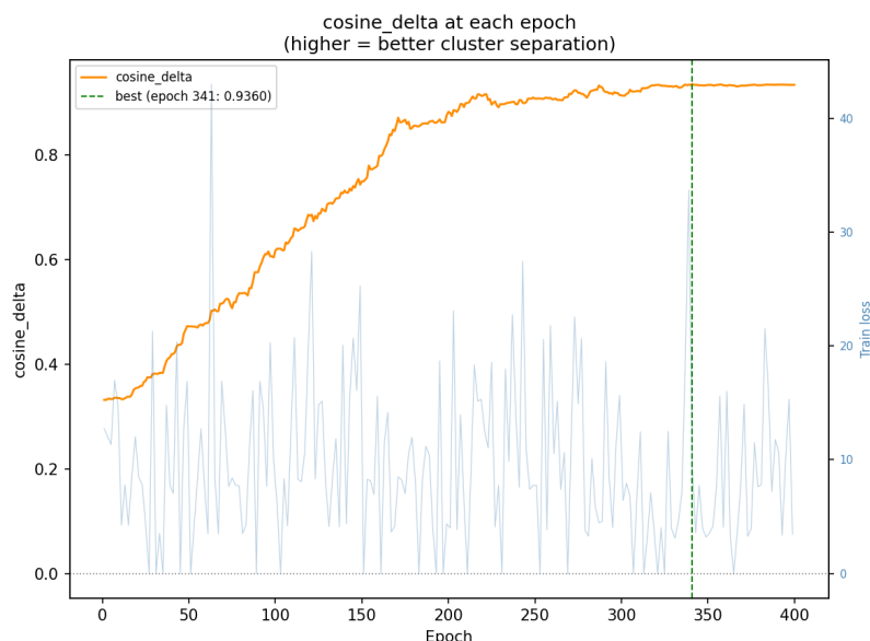
Figura 9.6: Evolución del cosine_delta (eje izquierdo) y de la pérdida de Negative Sampling (eje derecho) durante el entrenamiento de Word2Vec sobre el corpus ampliado.
