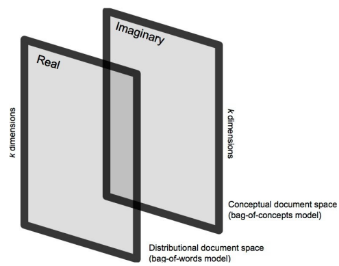
Figura 6.5: Esquema del espacio documental complejo vectorial unificando la semántica distribucional y referencial en el espacio de Hilbert. Fuente: [51].
