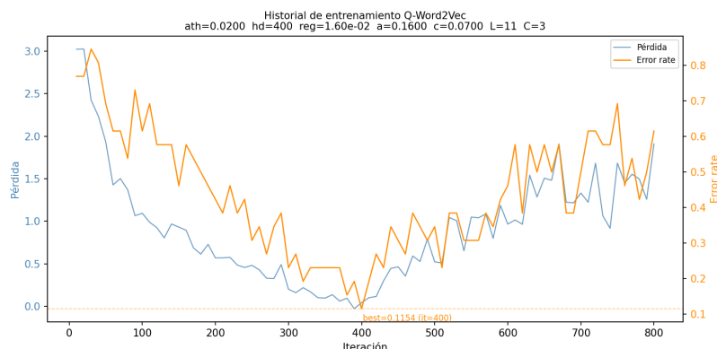
Figura 9.9: Evolución de la función de pérdida (eje izquierdo) y del error rate (eje derecho) durante el entrenamiento de QWord2Vec sobre el corpus ampliado.
