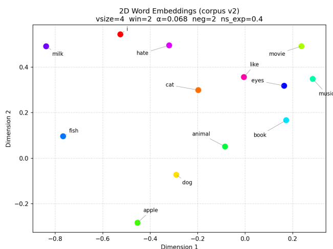
Figura 9.7: Visualización de los embeddings de Word2Vec obtenidos con el corpus ampliado, proyectados sobre las dos primeras dimensiones del espacio de embedding. Cada palabra se colorea según su clúster semántico de referencia.
