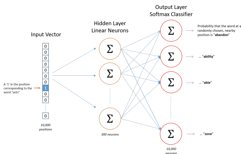
Figura 7.5: Arquitectura de la red neuronal del modelo Skip-gram. Fuente: [24].
