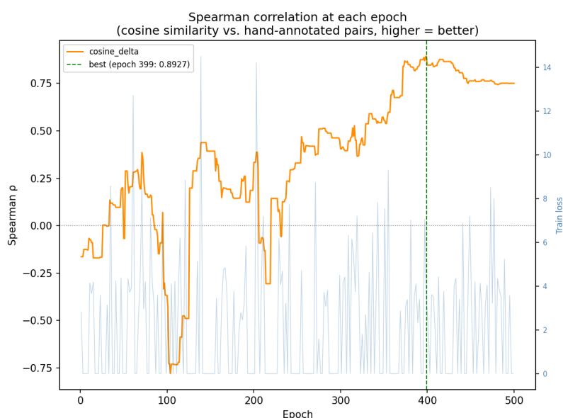
Figura 9.2: Evolución del cosine_delta (eje izquierdo, naranja) y del train loss (eje derecho, azul) a lo largo del entrenamiento de Word2Vec. La línea vertical verde indica la época en la que se registró el mejor checkpoint .
