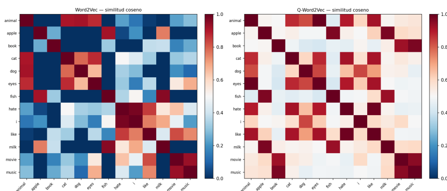
Figura 9.8: Matrices de similitud coseno para Word2Vec (izquierda) y QWord2Vec (derecha) entrenados con el corpus ampliado.
