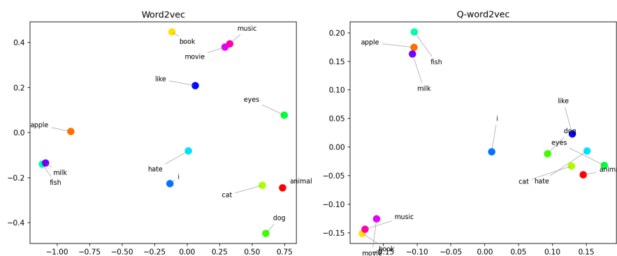
Figura 9.10: Comparación de los embeddings de Word2Vec (izquierda) y QWord2Vec (derecha) entrenados con el corpus ampliado. Para QWord2Vec se aplica PCA sobre las distribuciones de probabilidad de dimensión 2^4 = 16 .
