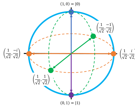
Figura 3.1: Visualización gráfica de la esfera de Bloch. Imagen obtenida de [45]
