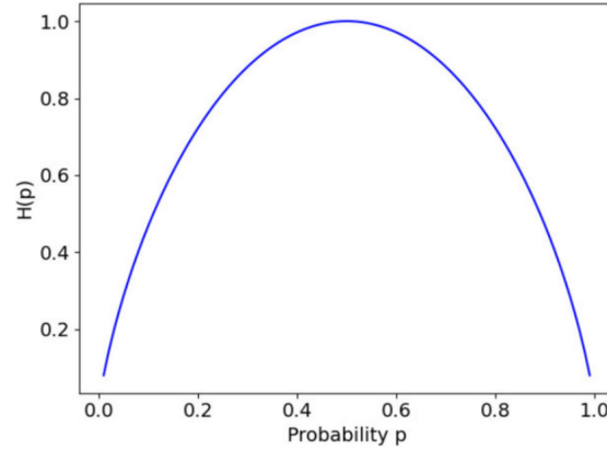
Figura 8.4: Entropía binaria H(p) , donde p denota la probabilidad de error empleada en este estudio. Fuente: [28].
