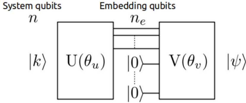
Figura 3.14: Estructura de QWord2Vec . Fuente: [34].
