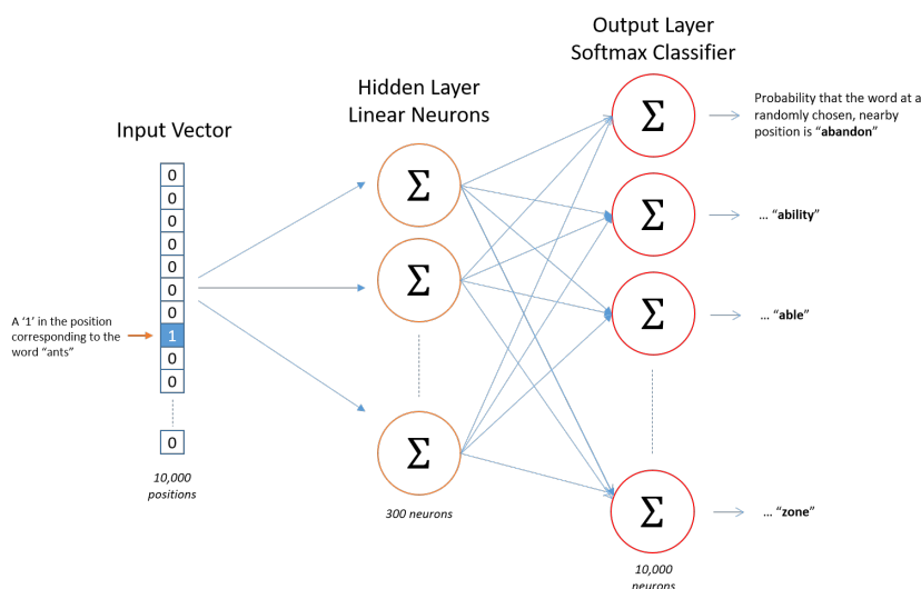
Figura 3.10: Arquitectura de la red neuronal del modelo Skip-gram. Fuente: [29].
