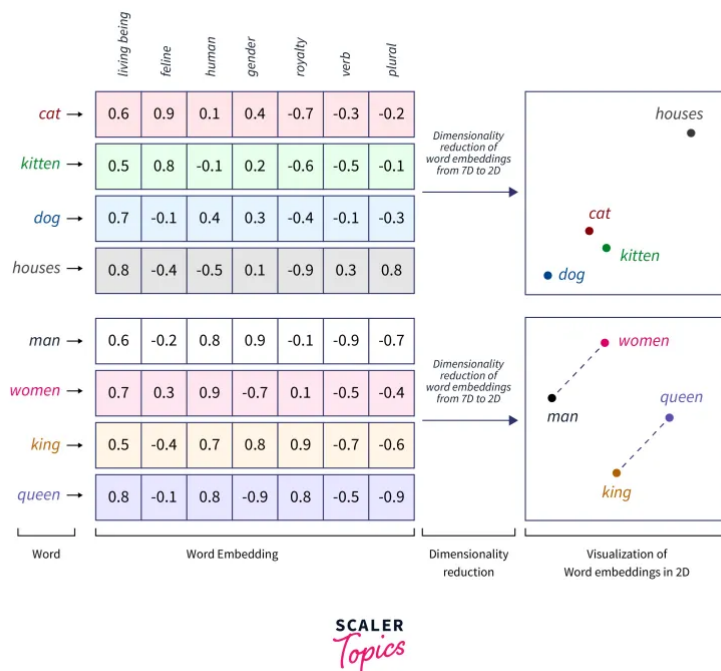
Figura 3.3: Representación visual de un modelo basado en conteos para generar embeddings de palabras. Fuente: [28].
