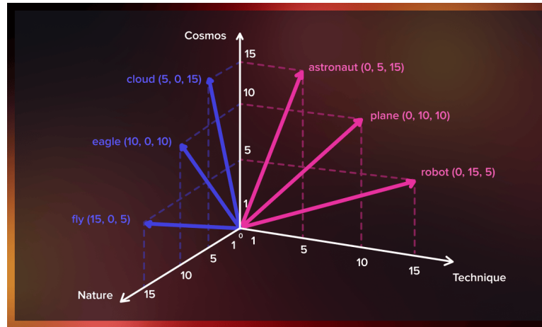
Figura 3.7: Representación vectorial de palabras en el espacio latente generado por Word2Vec. Fuente: [27].
