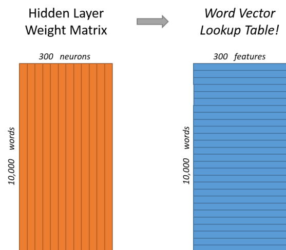
Figura 3.11: Matriz de pesos de la capa oculta del modelo Skip-gram: 10.000 filas (una por palabra del vocabulario) y 300 columnas (una por neurona oculta). Cada fila constituye el vector de representación de su palabra correspondiente. Fuente: [29].
