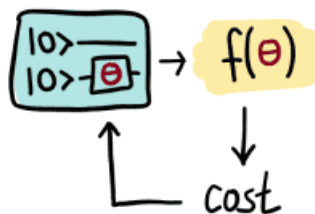
Figura 2.9: Coste de un Circuito Cuántico Variacional, imagen obtenida de: [36]
