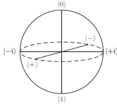
Figura 2.7: Imagen obtenida de [57]
