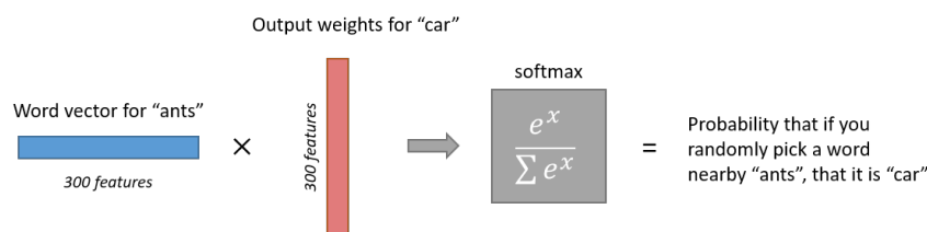
Figura 3.13: Cálculo de la salida de la neurona correspondiente a la palabra car en la capa softmax del modelo Skip-gram. Fuente: [29].
