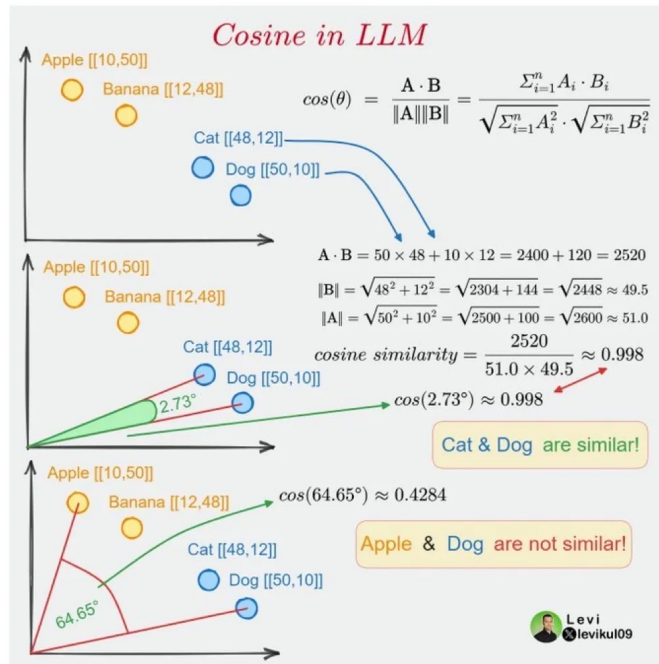
Figura 3.4: Ejemplo visual de la representación de vectores y su cercanía empleando la similitud coseno. Fuente: [25].
