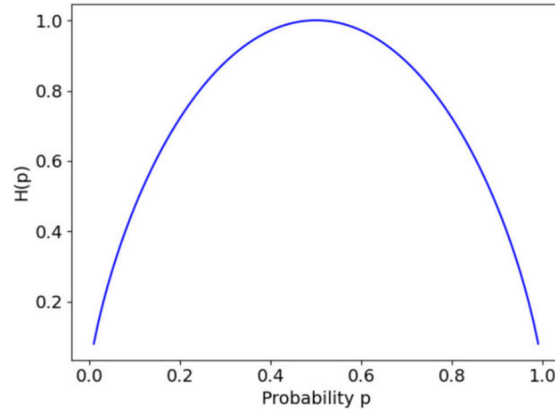
Figura 3.17: Entropía binaria H(p) , donde p denota la probabilidad de error empleada en este estudio. Fuente: [34].
