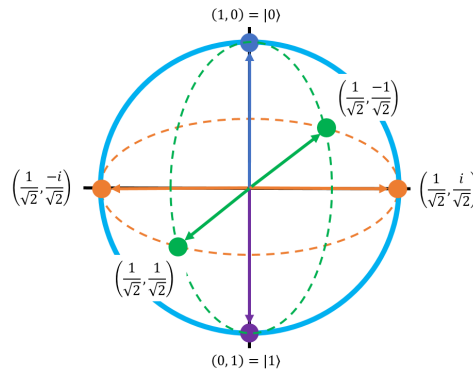
Figura 2.6: Visualización gráfica de la esfera de Bloch. Imagen obtenida de [52]
