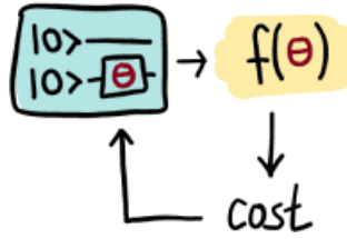
Figura 2.9: Coste de un Circuito Cuántico Variacional, imagen obtenida de: [61]
