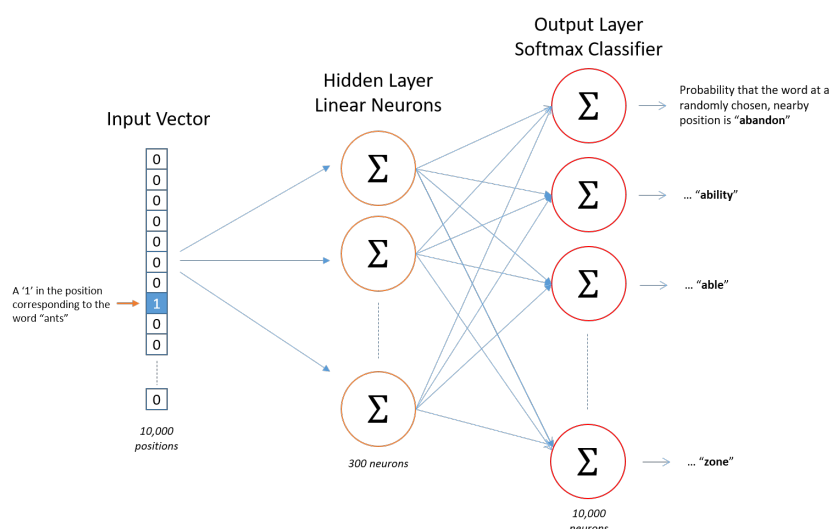
Figura 7.5: Arquitectura de la red neuronal del modelo Skip-gram. Fuente: [25].
