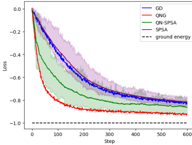
Figura 8.5: Comparativa de los algoritmos de optimización GD, SPSA, QNG y QN-SPSA en términos de convergencia y coste computacional. Fuente: [10].
