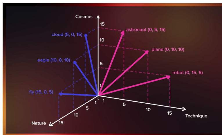
Figura 7.2: Representación vectorial de palabras en el espacio latente generado por Word2Vec. Fuente: [24].
