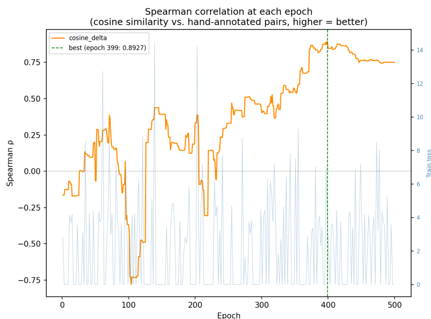
Figura 9.2: Evolución del cosine_delta (eje izquierdo, naranja) y del train loss (eje derecho, azul) a lo largo del entrenamiento de Word2Vec . La línea vertical verde indica la época en la que se registró el mejor checkpoint .
