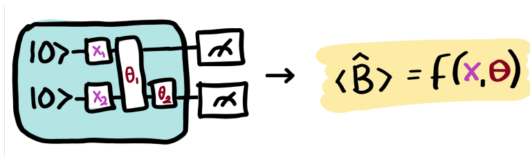
Figura 2.10: Circuito variacional cuántico con parámetros modificables \theta y no modificables x . Imagen obtenida de: [36]
