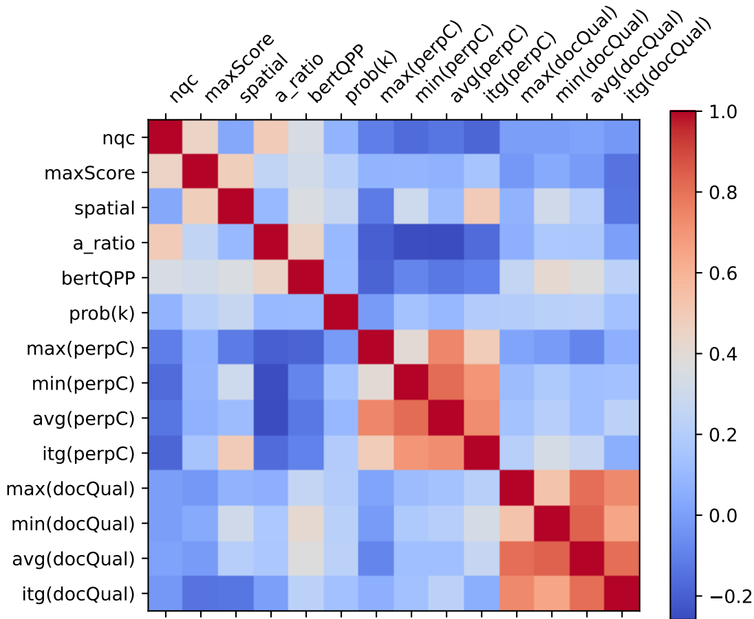
dl_bm25_5
