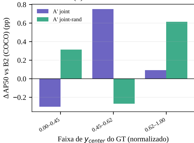
(b) Ganho estratificado
