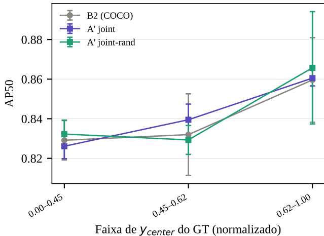
(a) AP50 por faixa vertical (medium)
