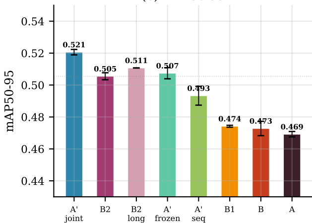
(b) mAP50-95
