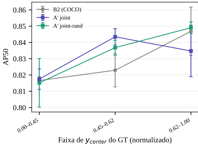
(a) AP50 por faixa vertical (todos os tamanhos)
