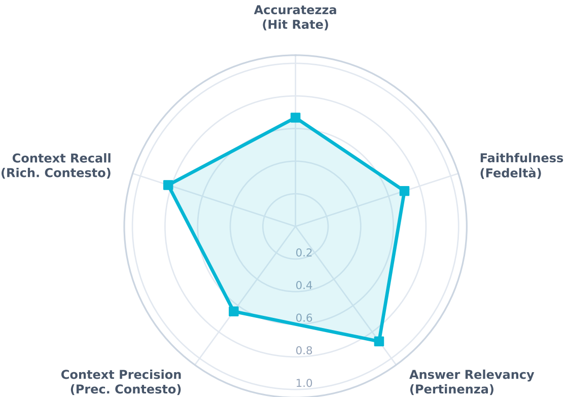
RAG Ibrido
