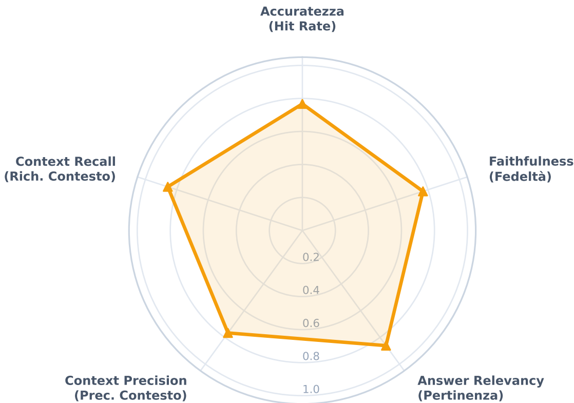
RAG Rerank
