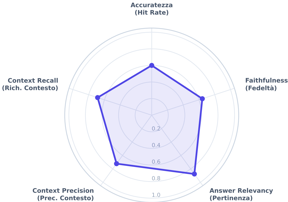
RAG Puro
