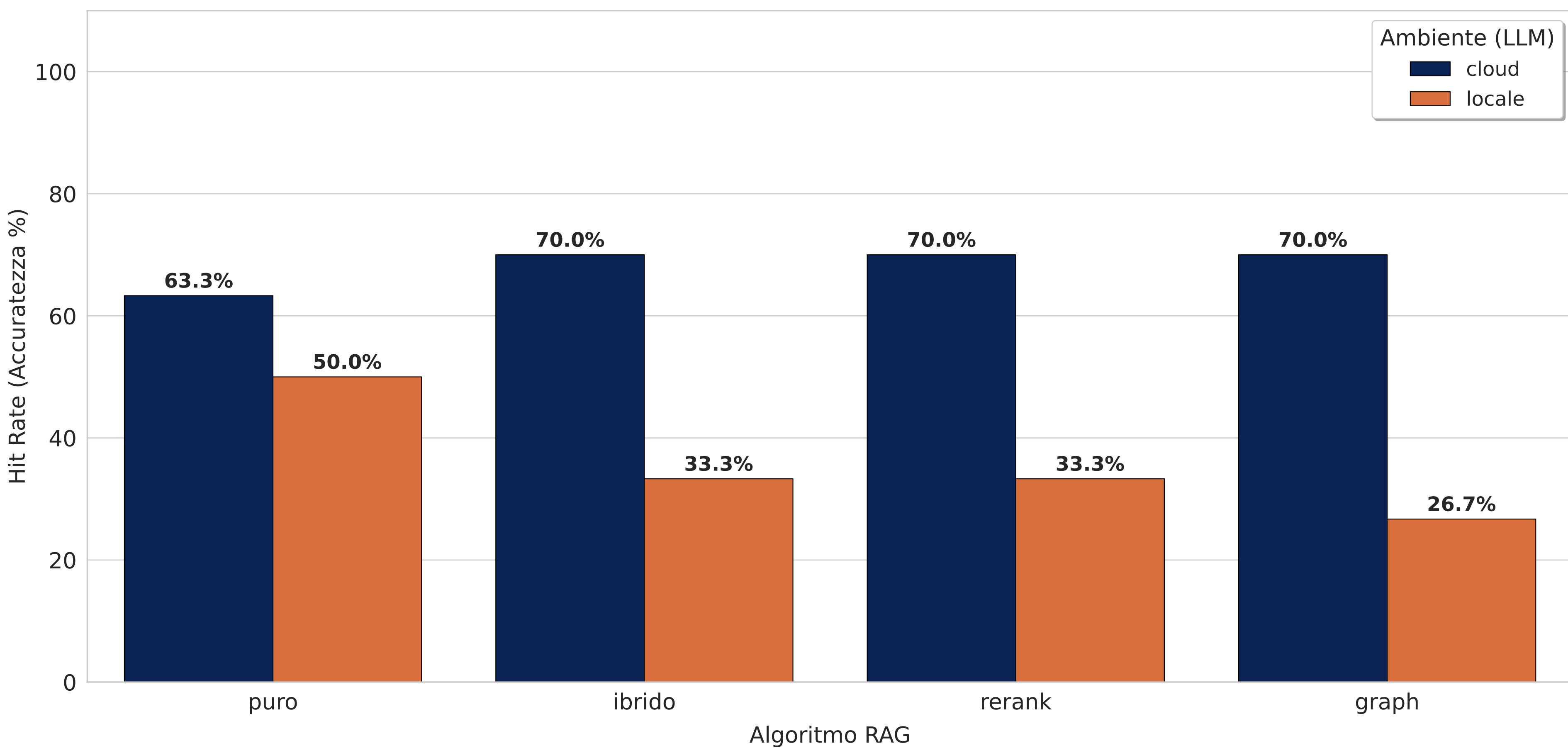
Accuratezza (Hit Rate %) - Italiano (it)
