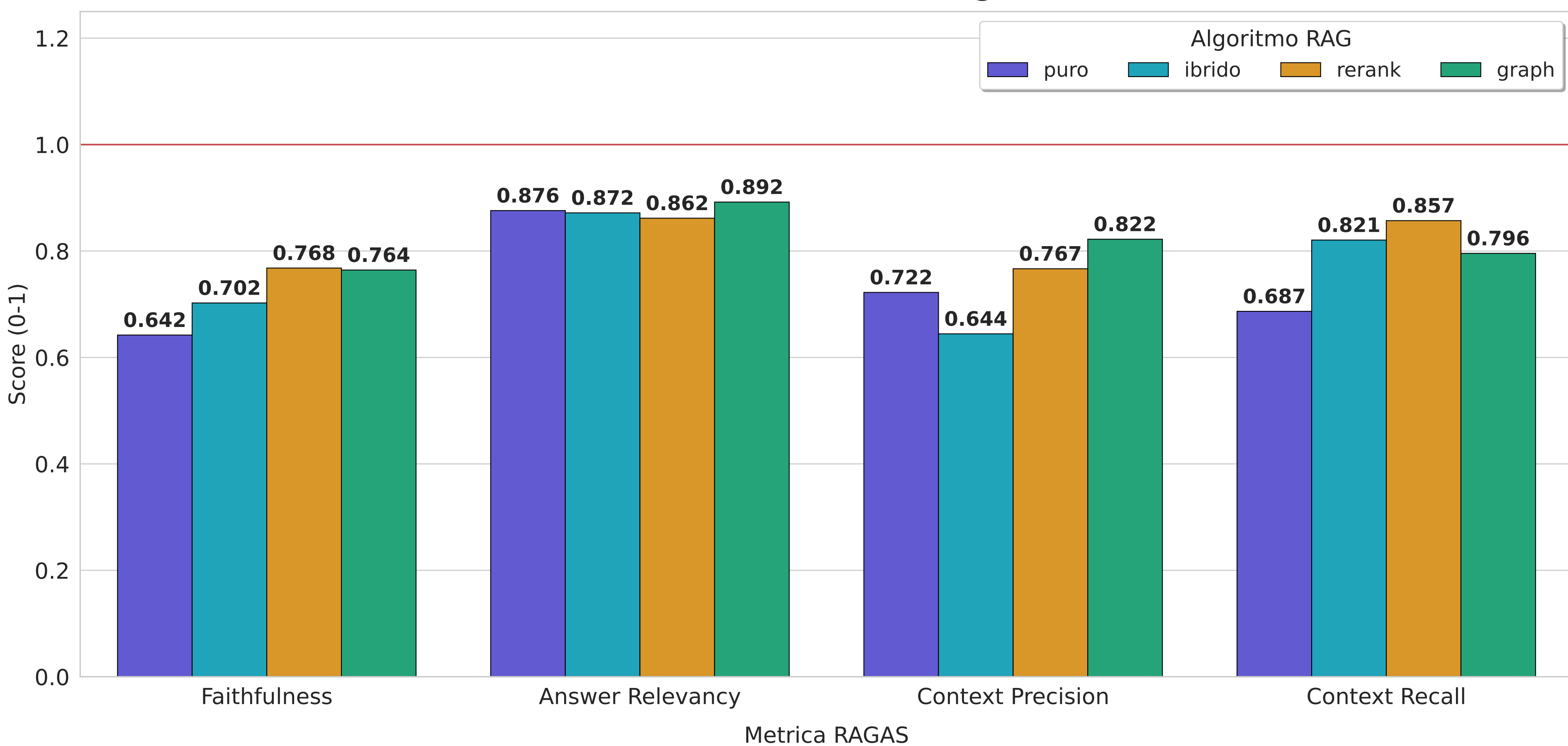
Metriche RAGAS in Cloud - Italiano (it)
