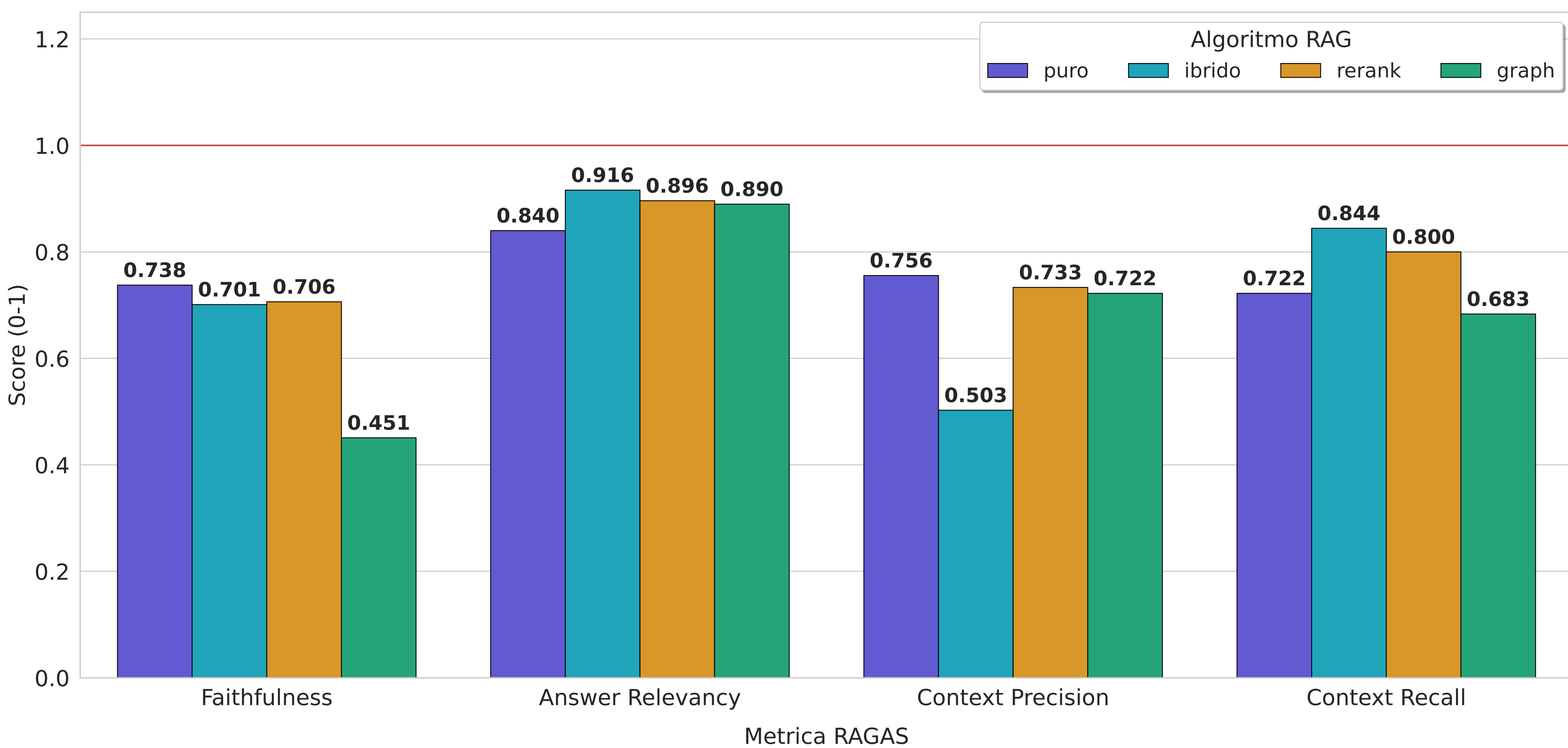
Metriche RAGAS in Cloud - Italiano (it)
