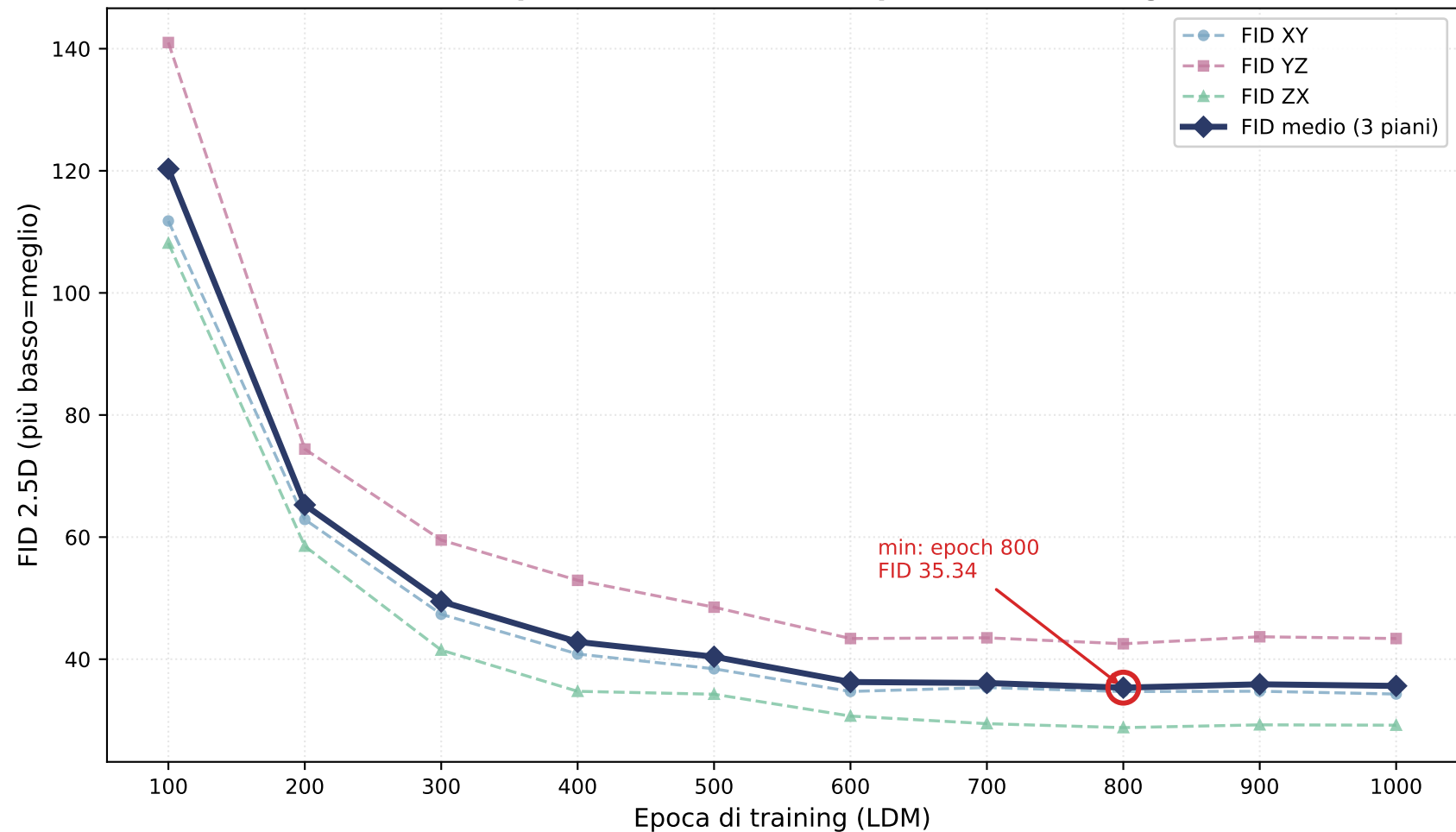
Selezione checkpoint LDM v4 - FID vs epoca (senza autoguidance)
