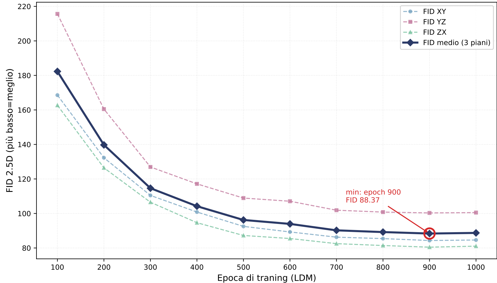
Evoluzione del FID durante il training dell'LDM
