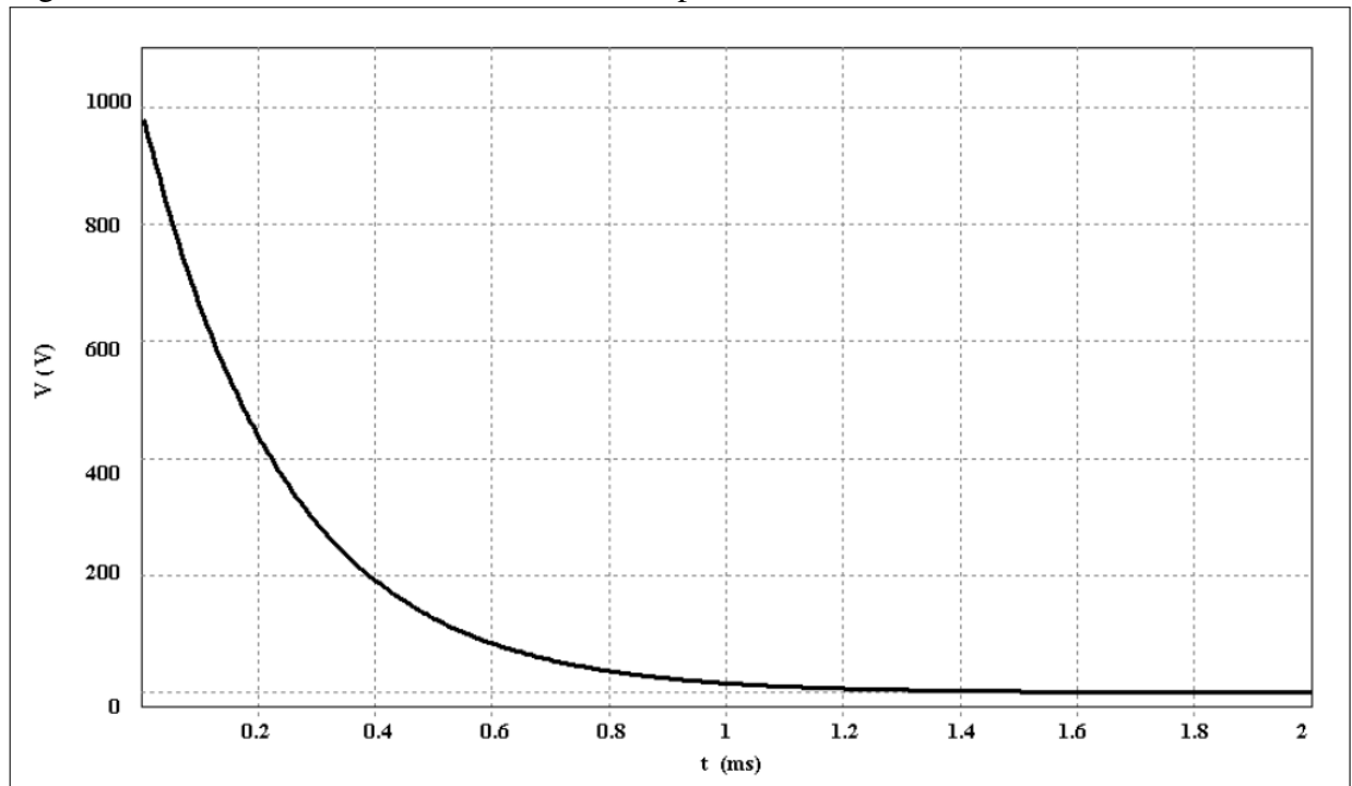
Figura 4 – Gráfico de tensão considerando a impedância humana
